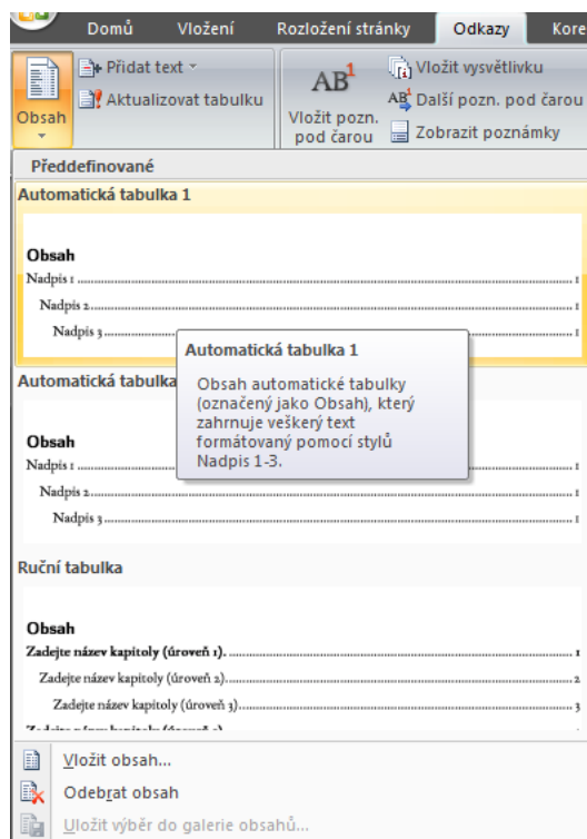
Obr. 19: Generování obsahu
