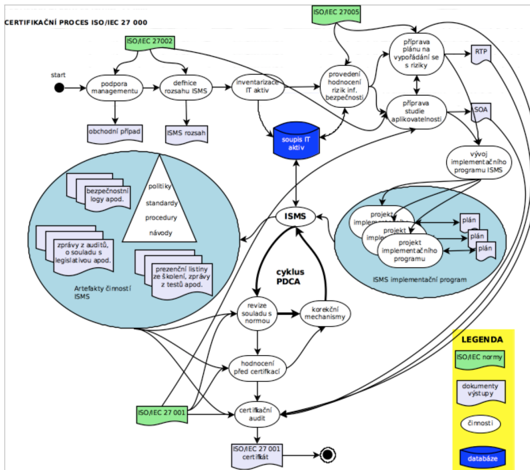
Obrázek 2.1: Certifikační proces ISMS (adaptováno z [43])
