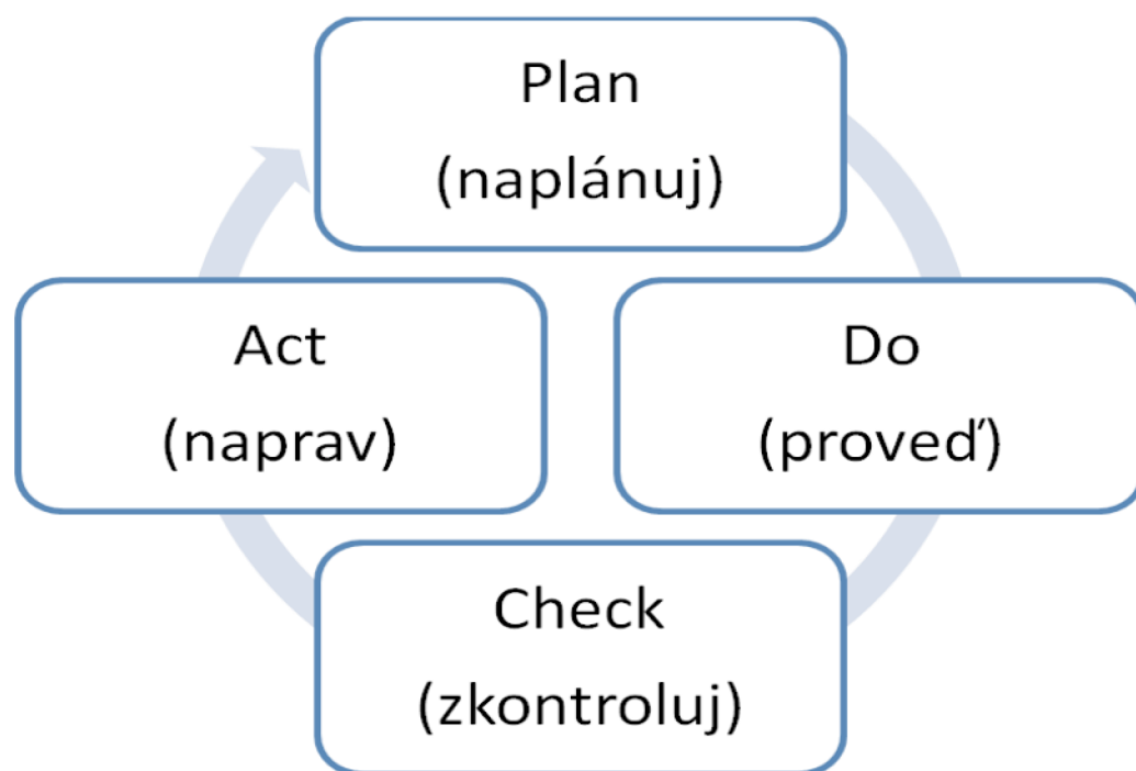
Obrázek 2.2: PDCA princip
