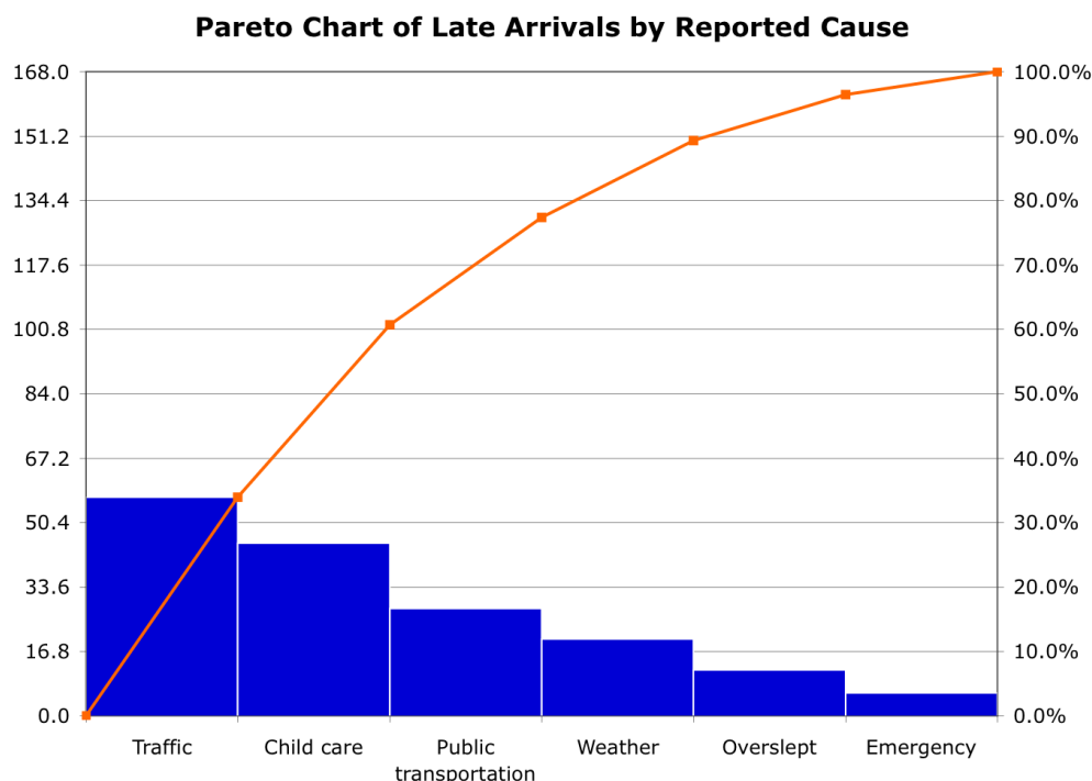
Obrázek 4.7: Paretův graf (převzato z [48])
