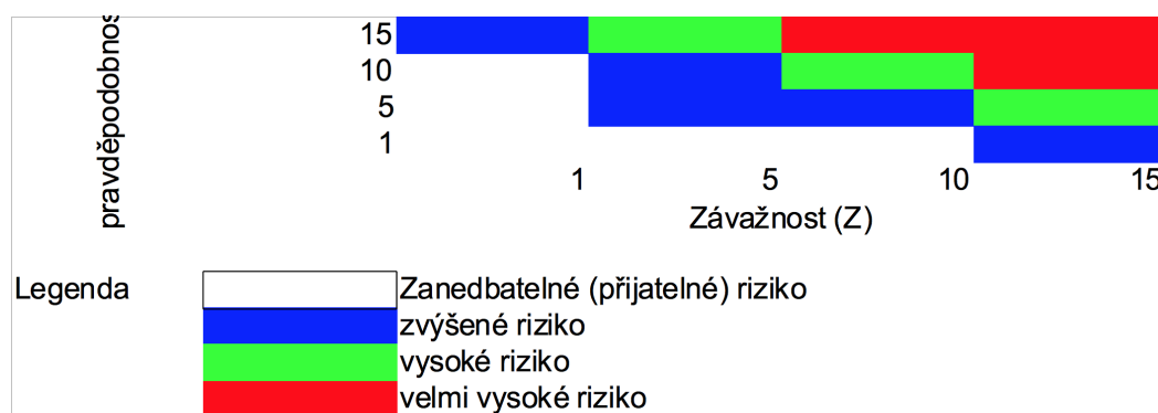
Obrázek 2.4: Matice rizik
