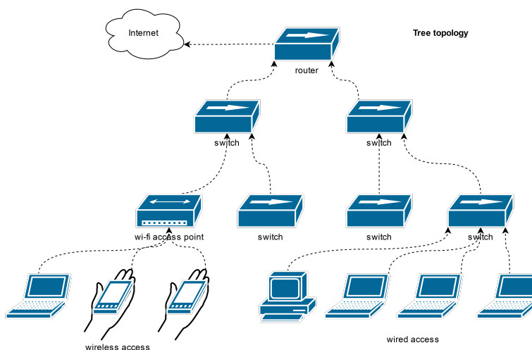
Obrázek 5.4: Stromová (hybridní) topologie
