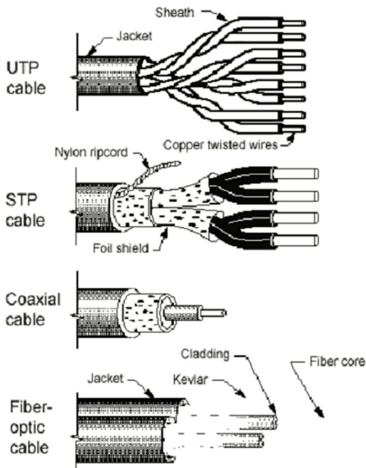
Obrázek 5.6: Nejčastěji používané typy kabeláže v počítačových sítích (převzato z [85])
