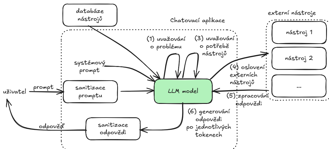
Obrázek 8.9: Schéma chatovací aplikace schopné pracovat v agentním režimu
