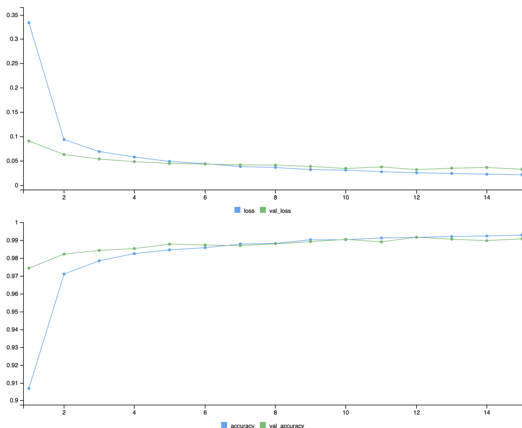
Obrázek 4.7: Proces adaptace konvoluční sítě
