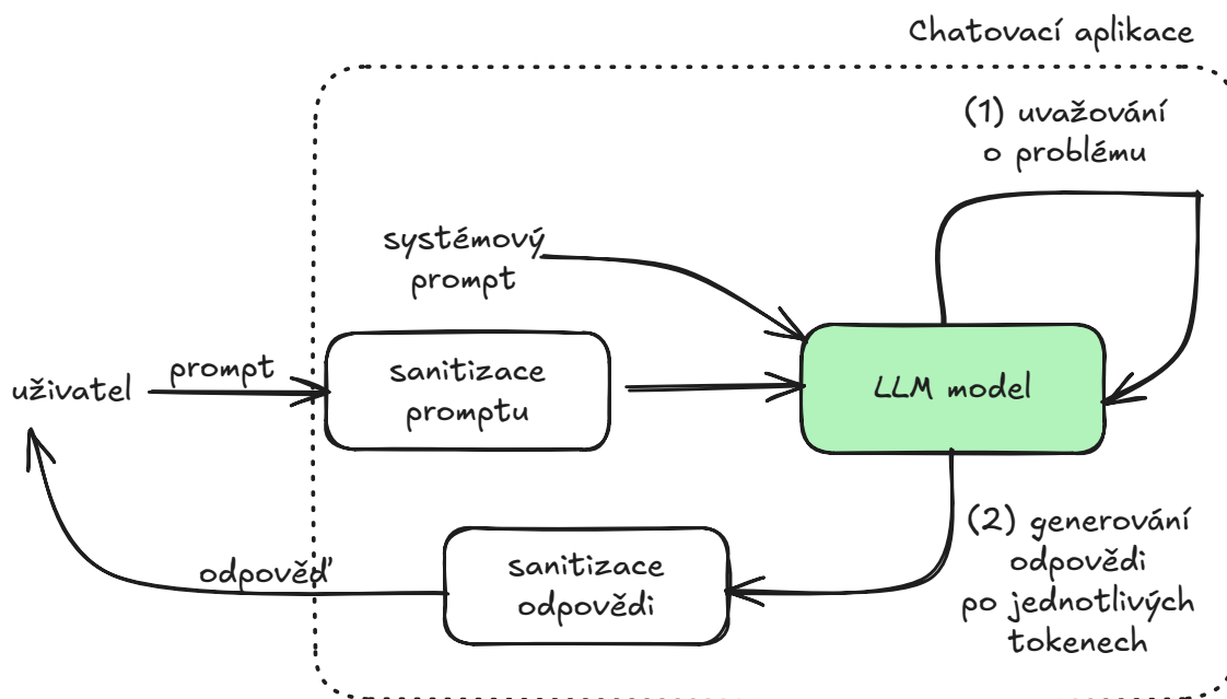
Obrázek 4.13: Struktura chatovací aplikace s modelem podporujícím CoT
