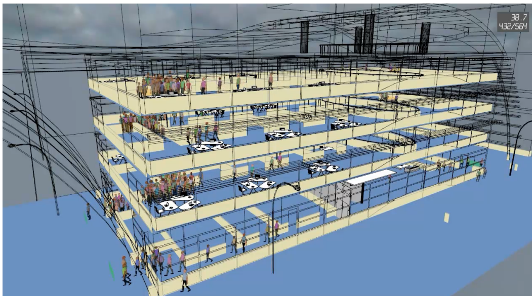
Obrázek 8.7: Simulace evakuace budovy v balíku SIMULEX (převzato z [52])
