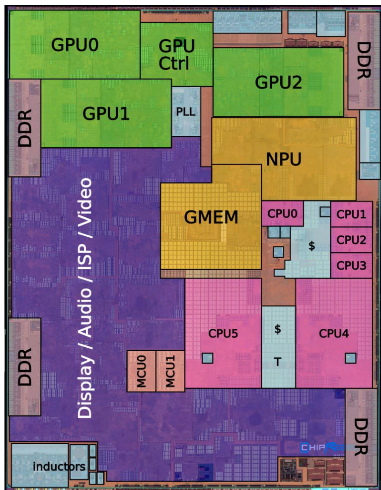
Obrázek 1.2: Analýza struktury čipu A11 Bionic (převzato z [82])
