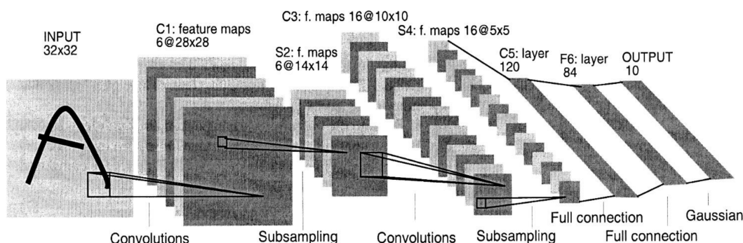
Obrázek 4.5: Konvoluční neuronová síť (převzato z [49])
