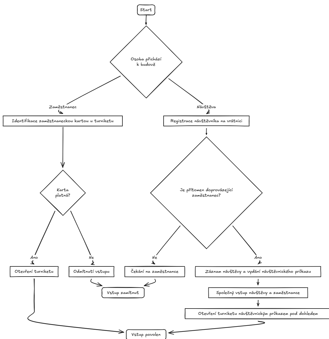
Obrázek 5.21: Diagram aktivit generovaný pomocí Mermaid v ExcaliDraw (vytvořeno pomocí Copilot)
