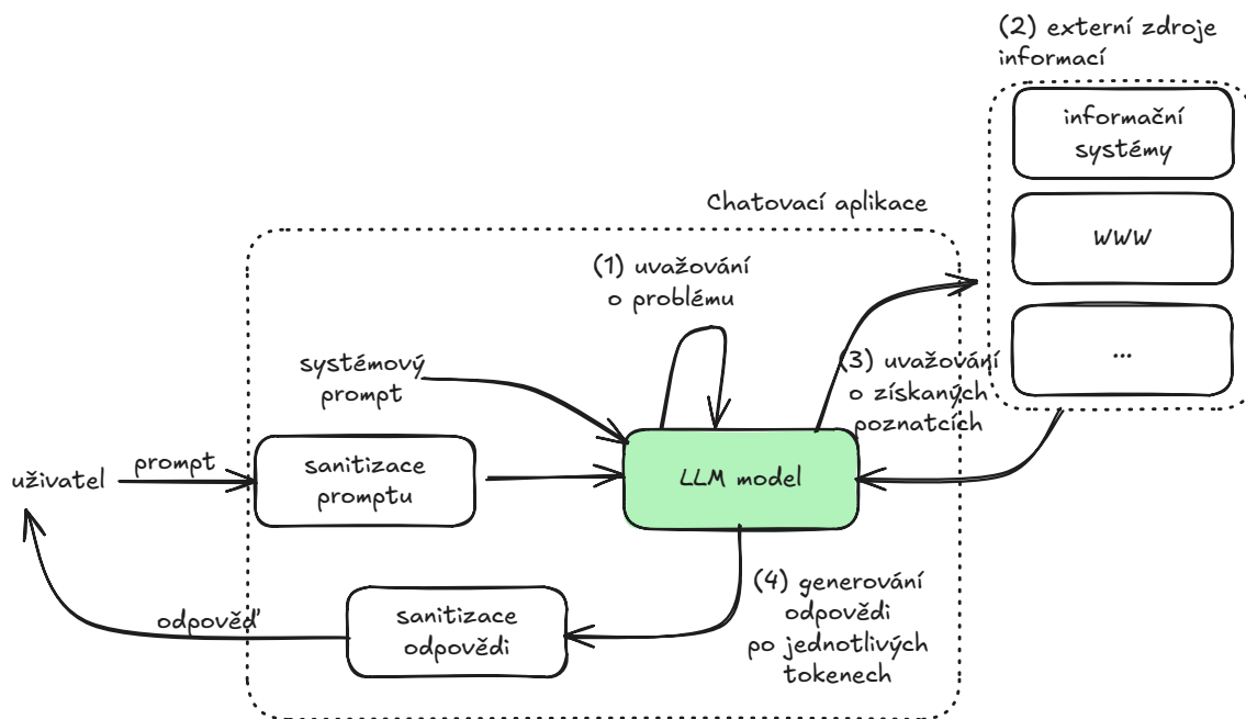
Obrázek 4.14: Struktura chatovací aplikace s modelem podporujícím CoT a RAG
