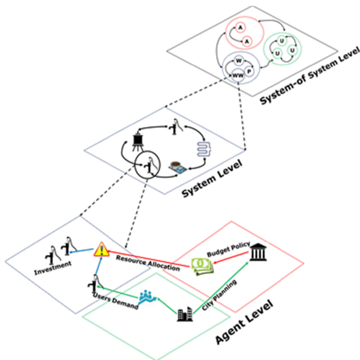
Obrázek 8.6: Rámec multiagentního systému pro abstrakci modelování kritické infrastruktury (převzato z [72])
