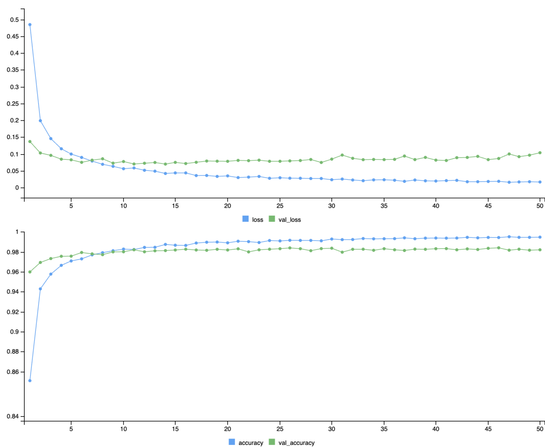
Obrázek 4.4: Proces adaptace klasické neuronové sítě v Keras pro MNist dataset
