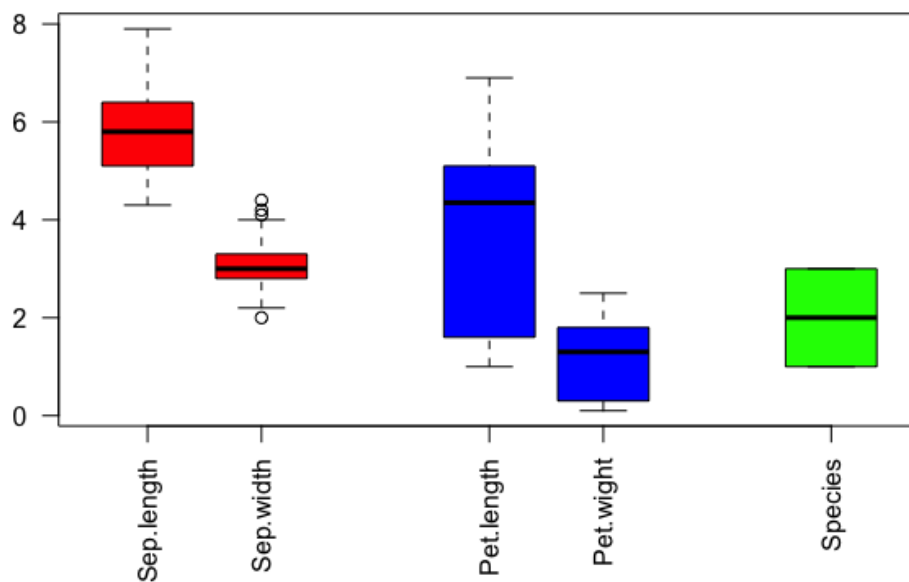
Obrázek 2.7: Délka listu dataset iris (boxplot)
