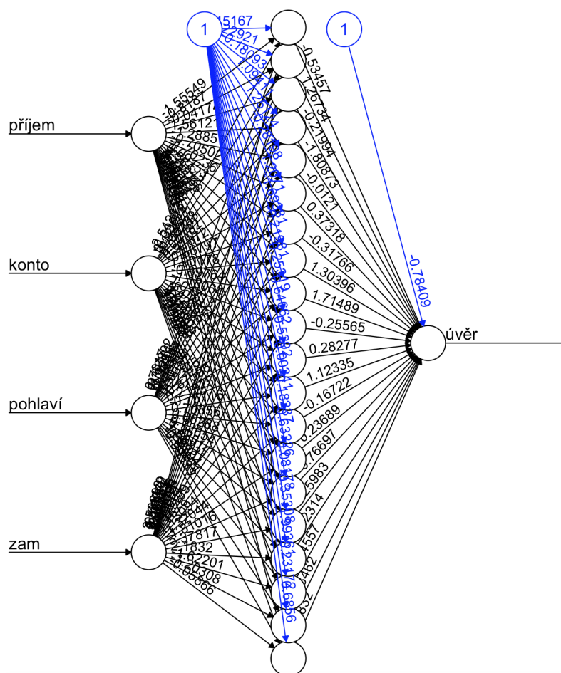
Obrázek 3.10: Klasifikace klientů banky neuronovou sítí
