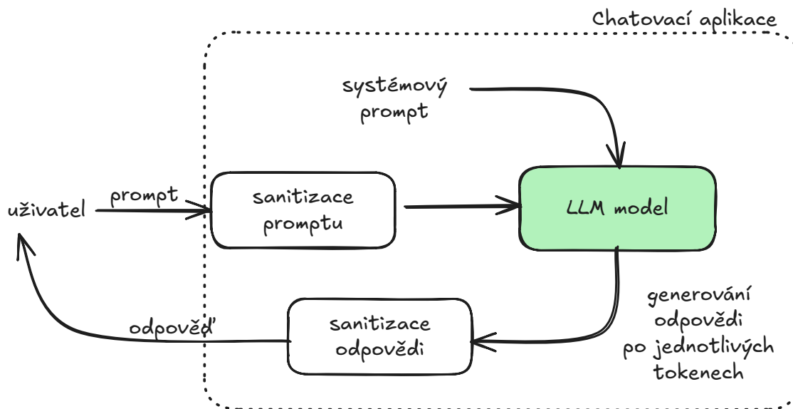
Obrázek 4.12: Základní struktura chatovací aplikace - model bez jakýchkoliv zvláštních schopností
