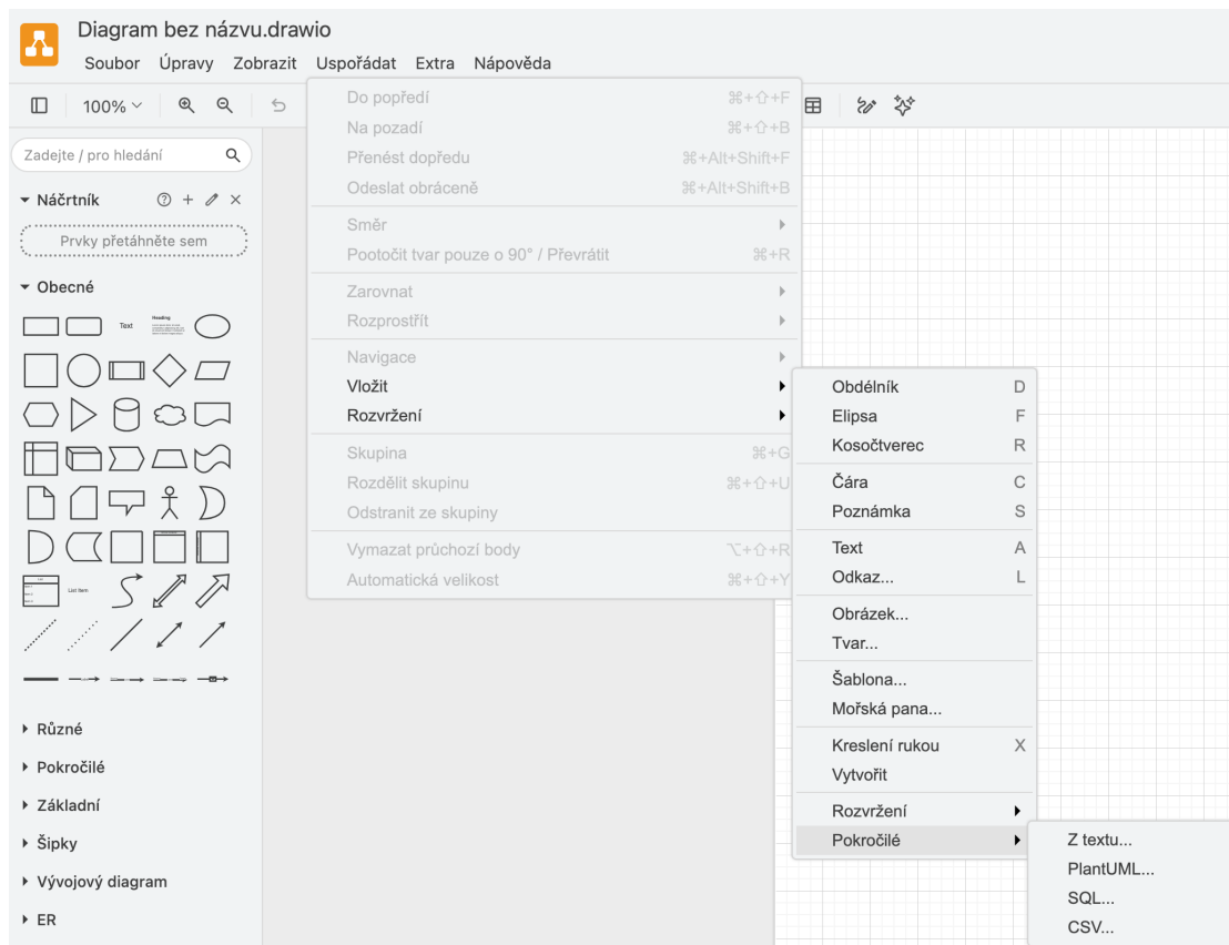
Obrázek 5.18: Import diagramu ve formátu Mermaid do nástroje Draw.io
