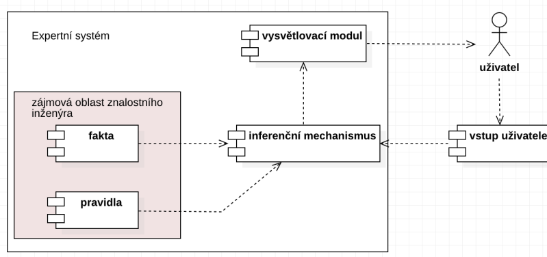
Obrázek 6.1: Struktura expertního systému
