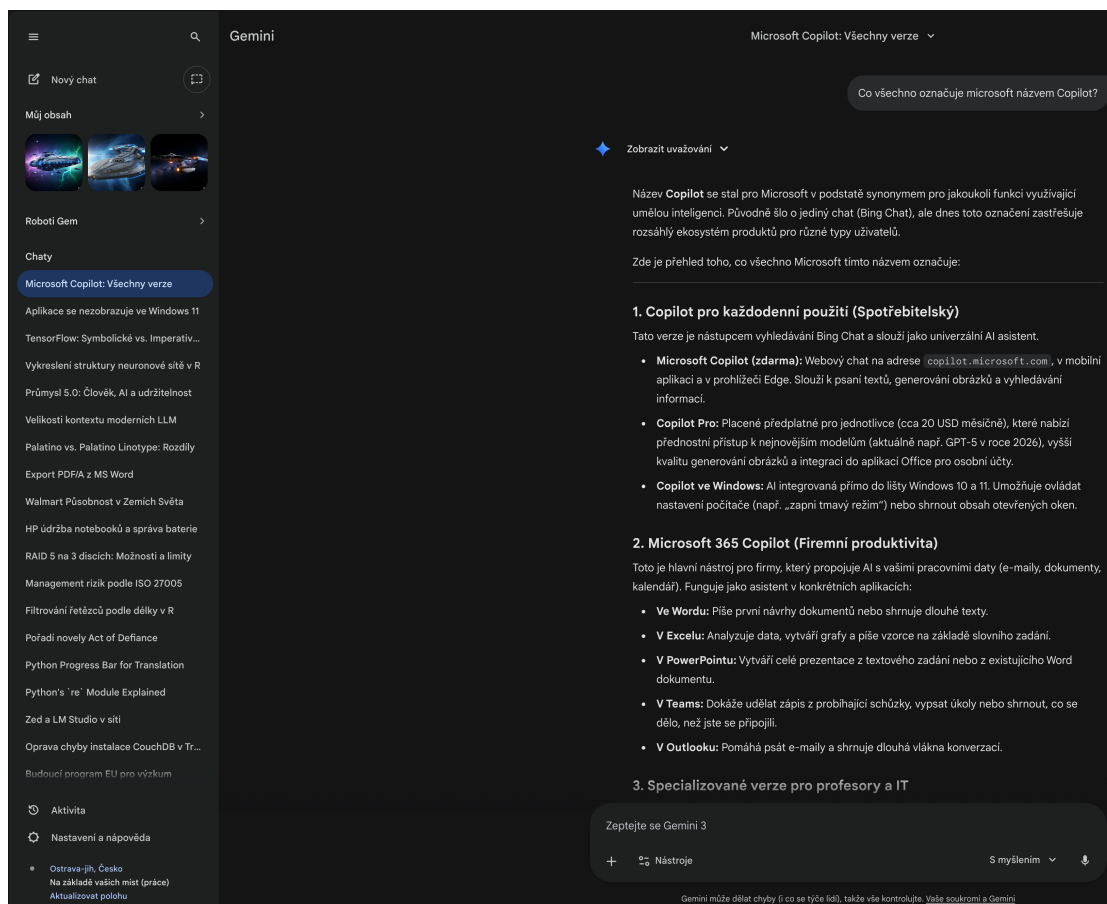
Obrázek 4.9: Google Gemini
