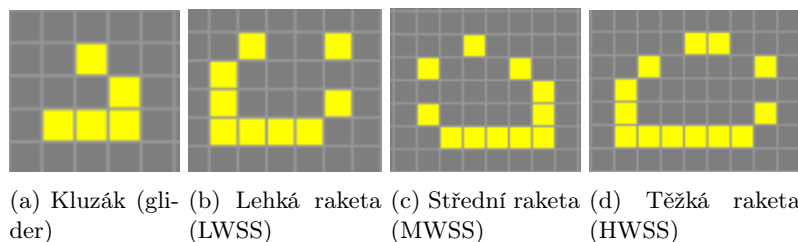
Obrázek 7.5: Conwayova hra života - pohybující se struktury
