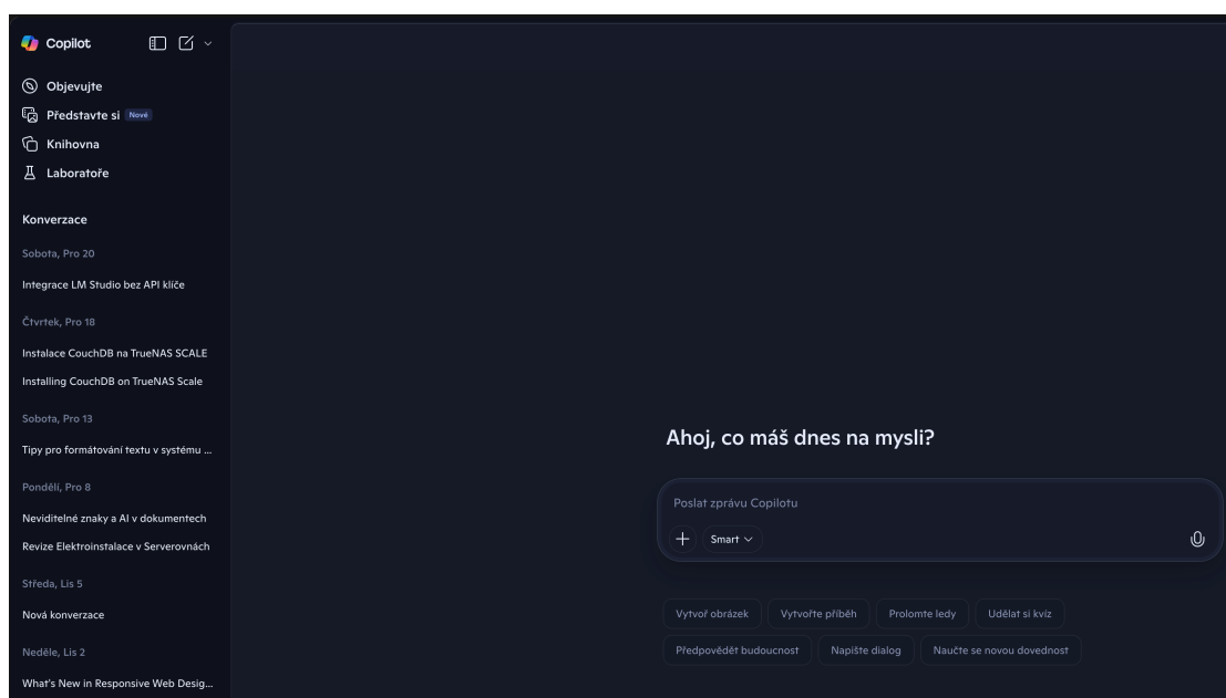
Obrázek 4.8: MS Copilot
