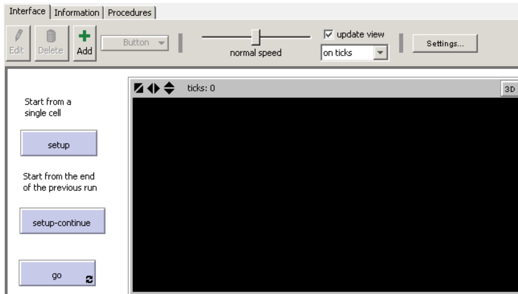
Obrázek 7.14: GUI NetLogo
